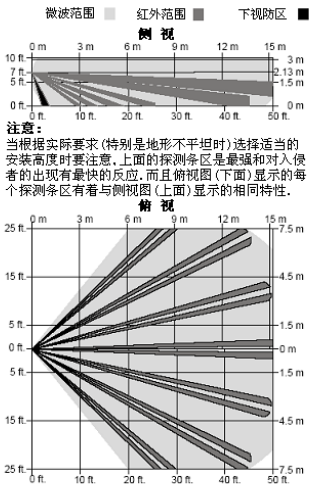
图 1- 探测范围
